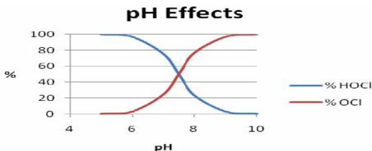
HOCL 与 PH 的关系图
