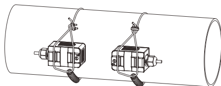
钢丝绳固定 >DN500
