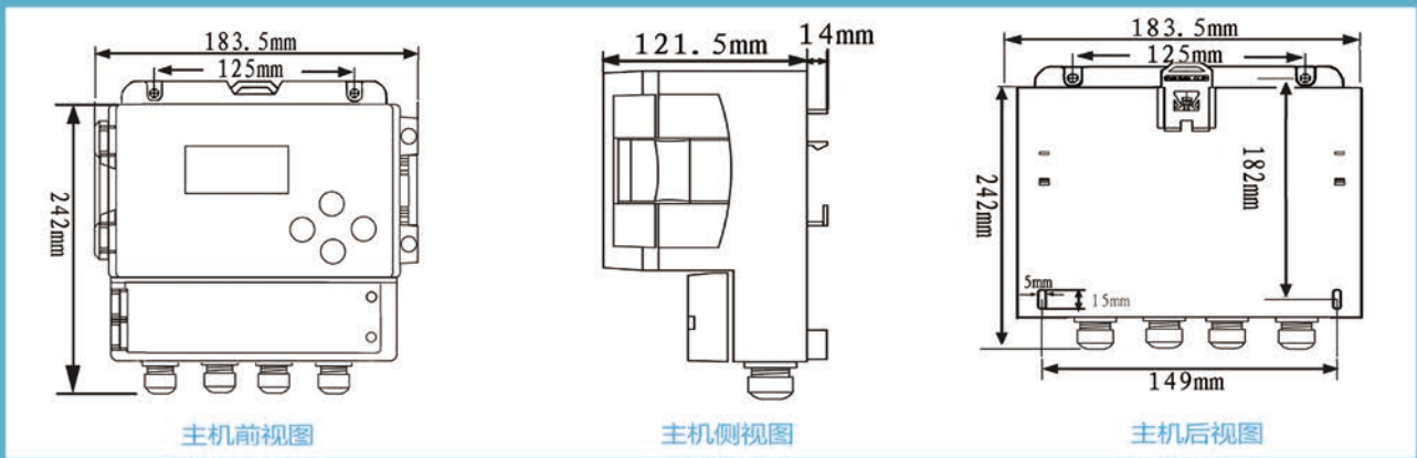
壁挂主机尺寸图示
