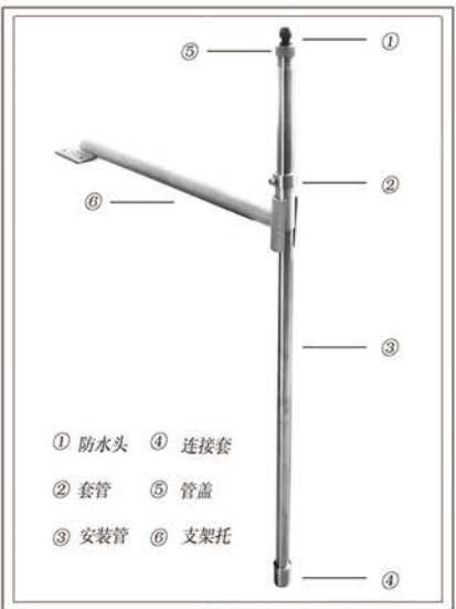
超声波液位计安装支架不锈钢304
