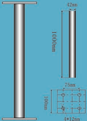
仪表箱底座
